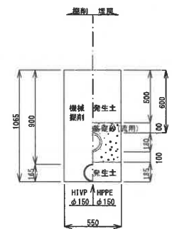
9 本設 (未舗装) H=0.60m
