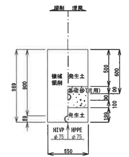
11 本設 (未舗装) H=0.60m
