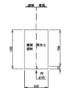
38 仮設 (未舗装) H=0.79m
