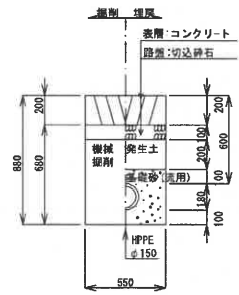
6 本設 (Co舗装) H=0.60m
