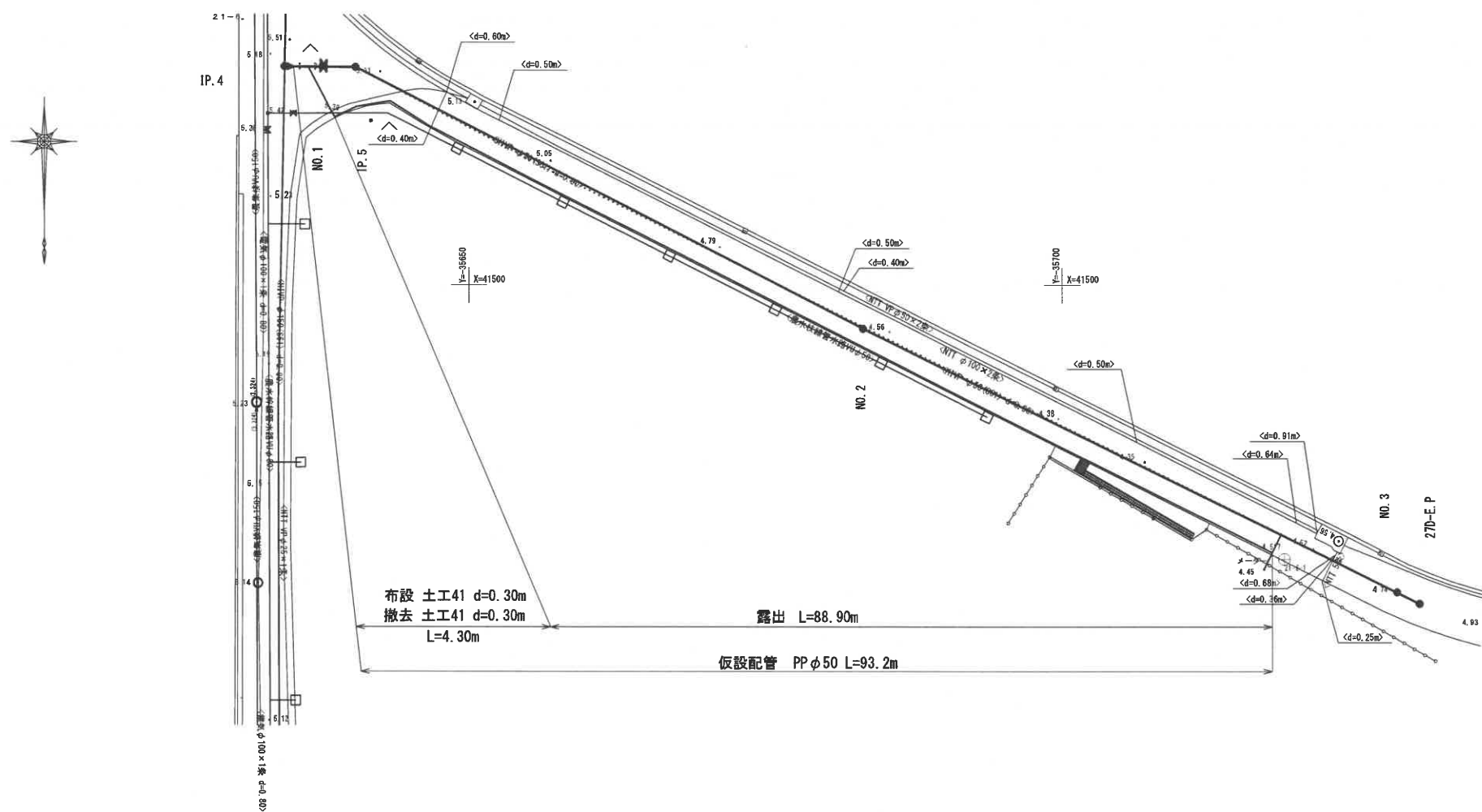
仮設配管平面図 (27号線D2)
