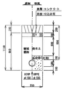
2 本設 (Co舗装) H=0.90m
