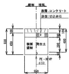
13 ドレン設置 (Co舗装) H=0.49m
