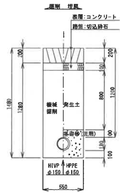
1 本設 (Co舗装) H=1.20m
