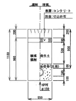
5 本設 (Co舗装) H=0.90m
