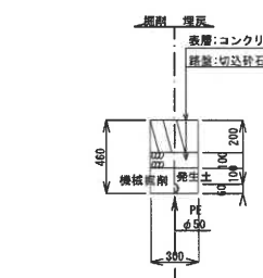
41 仮設給水 (舗装) H=0.30m
