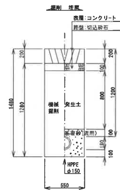
4 本設 (Co舗装) H=1.20m
