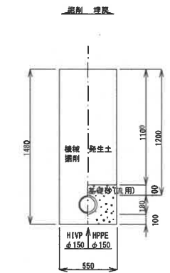
7 本設 (未舗装) H=1.20m
