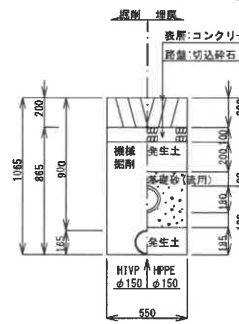
3 本設 (Co舗装) H=0.60m
