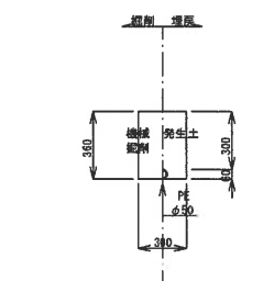
40 仮設給水 (未舗装) H=0.30m
