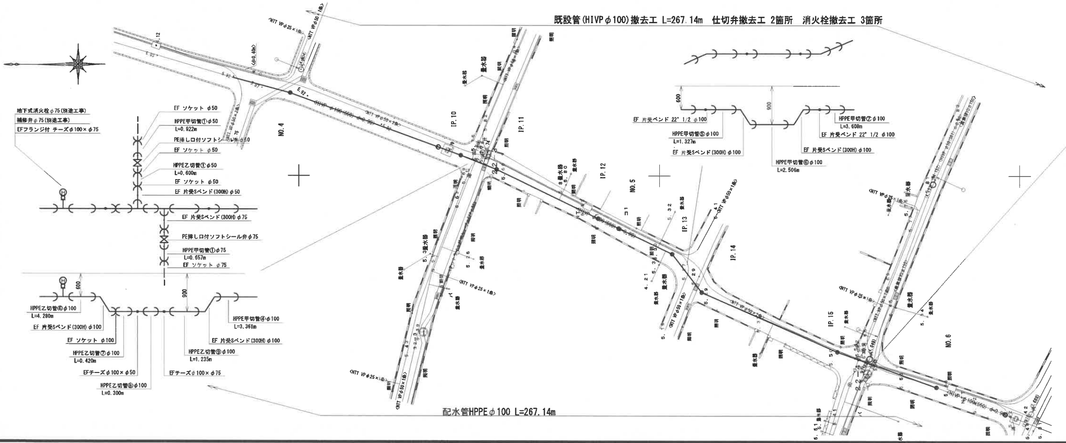
配水管平面図(5号線 2/3)
