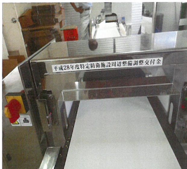
4 金属検出オートチェッカー
