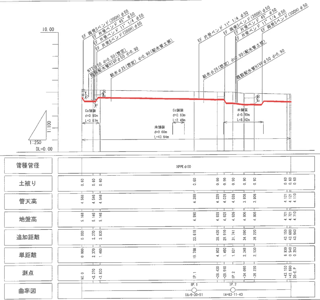
配水管縦断図(25号線) V=1:100 H=1:250
