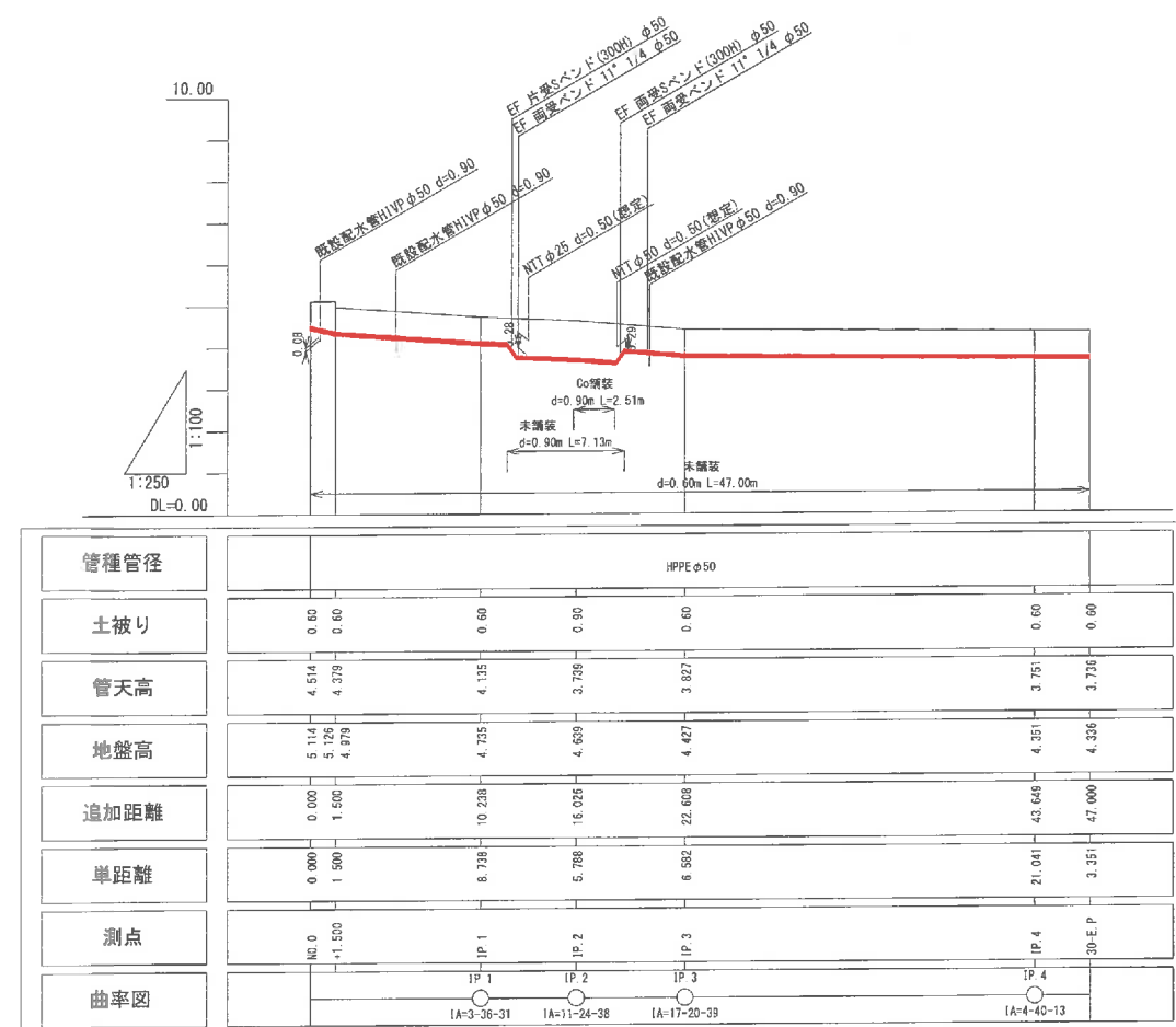
配水管縦断面図(30号線) V=1:100 H=1:250
