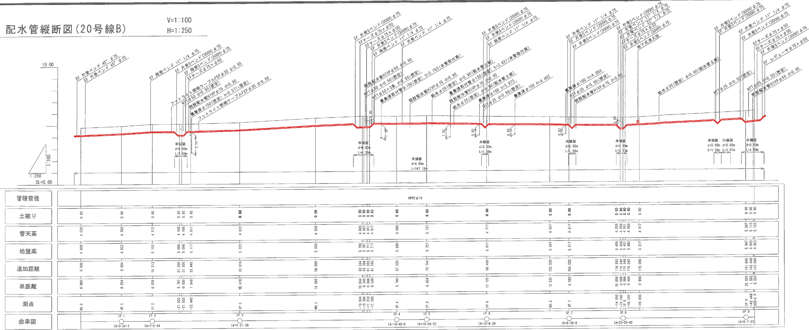
配水管平面図(20号線B)
