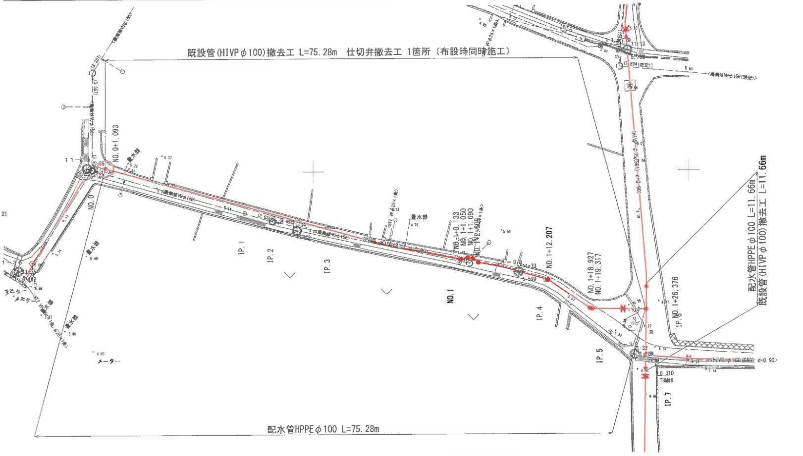
配水管平面図(13号線B 1/2)
