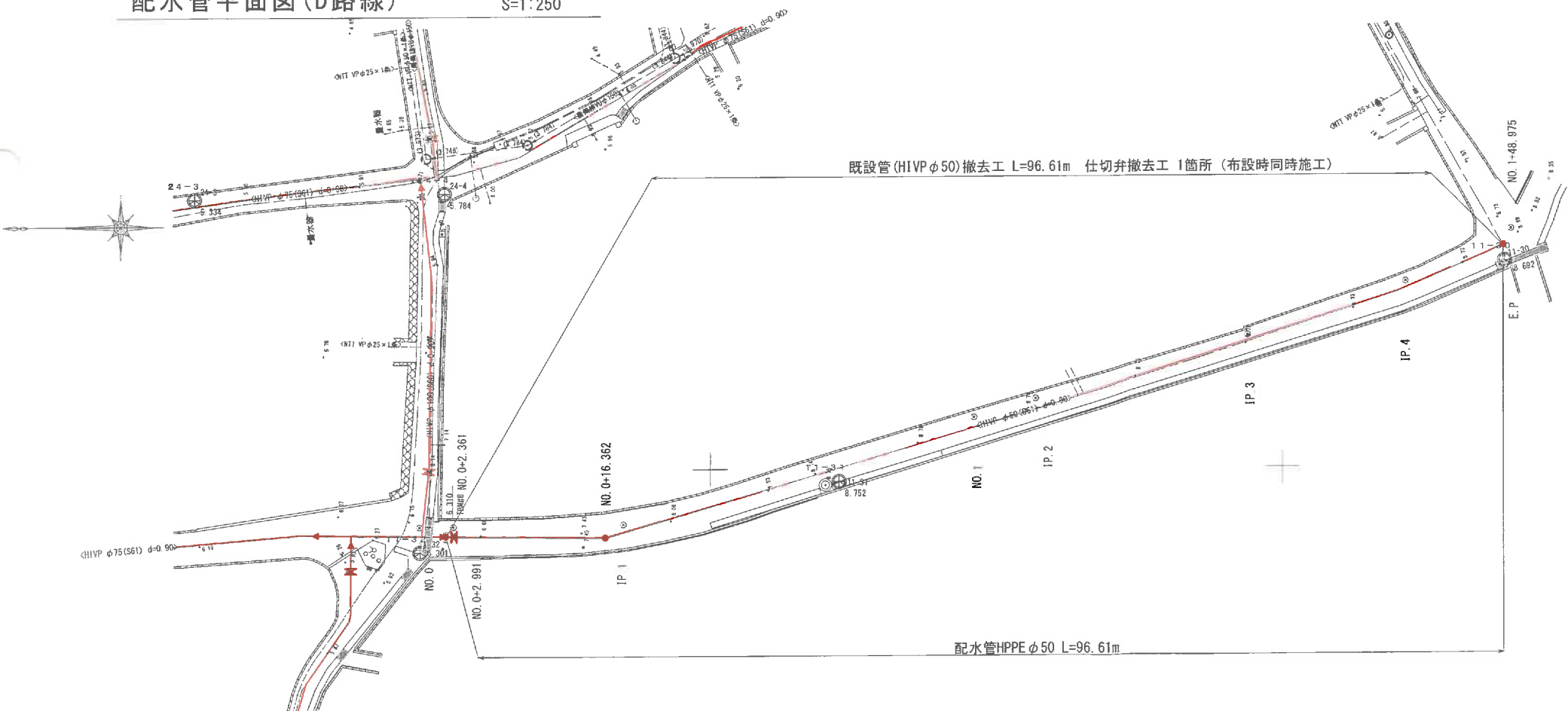
配水管平面図(D路線) S=1:250
