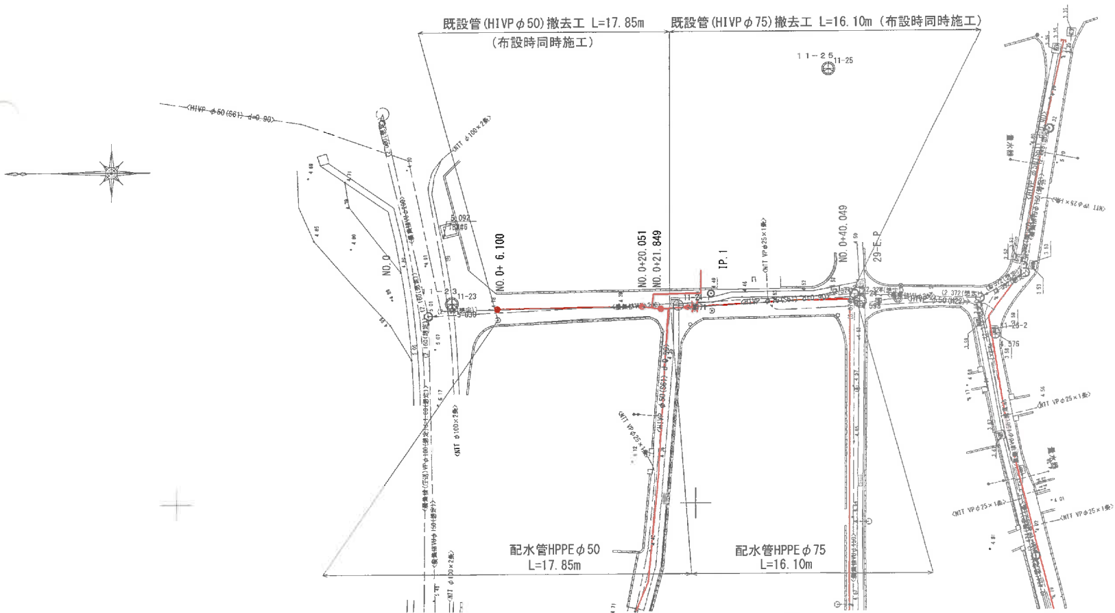
配水管平面図(29号線)
