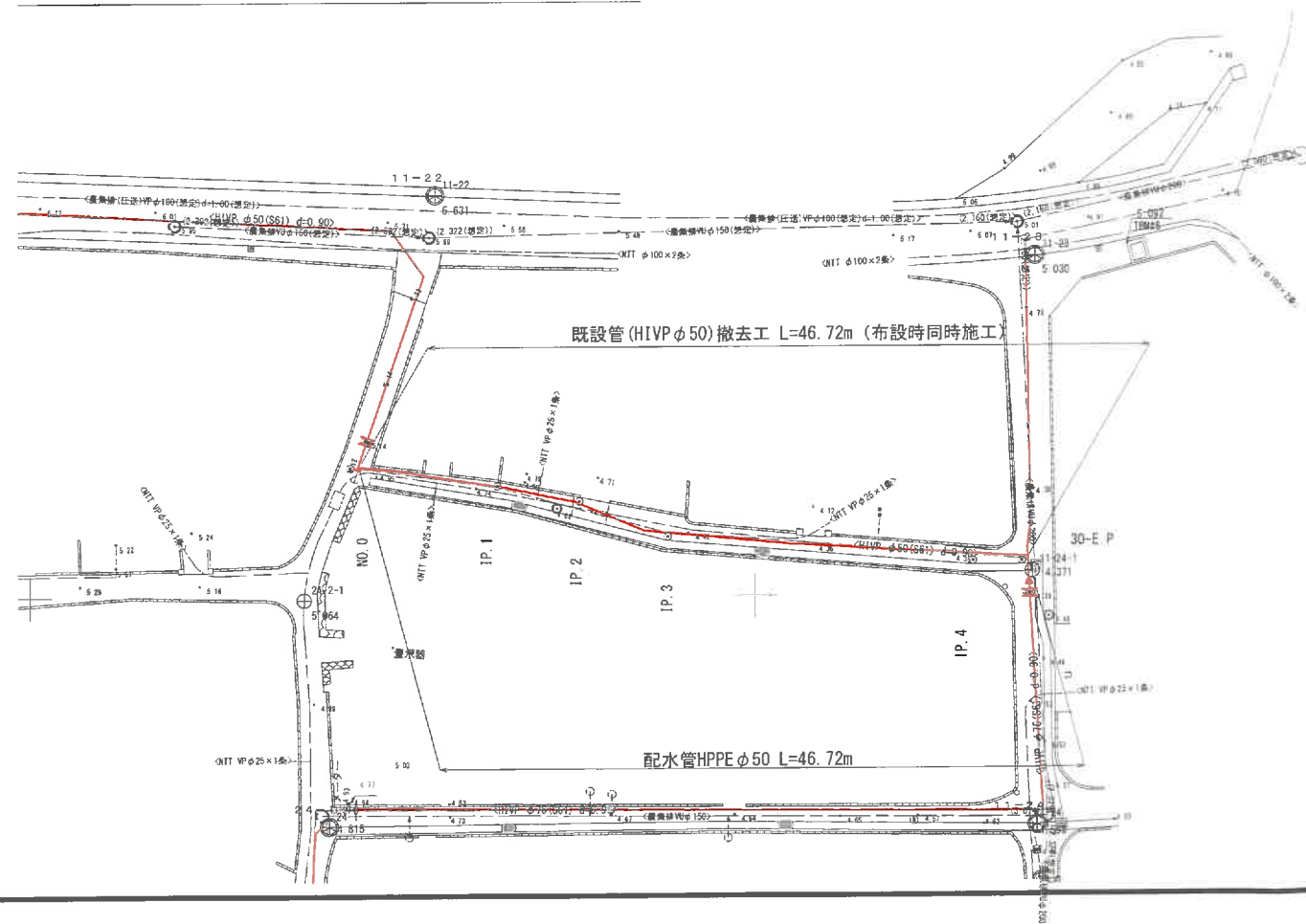
配水管平面図(30号線) S=1:250
