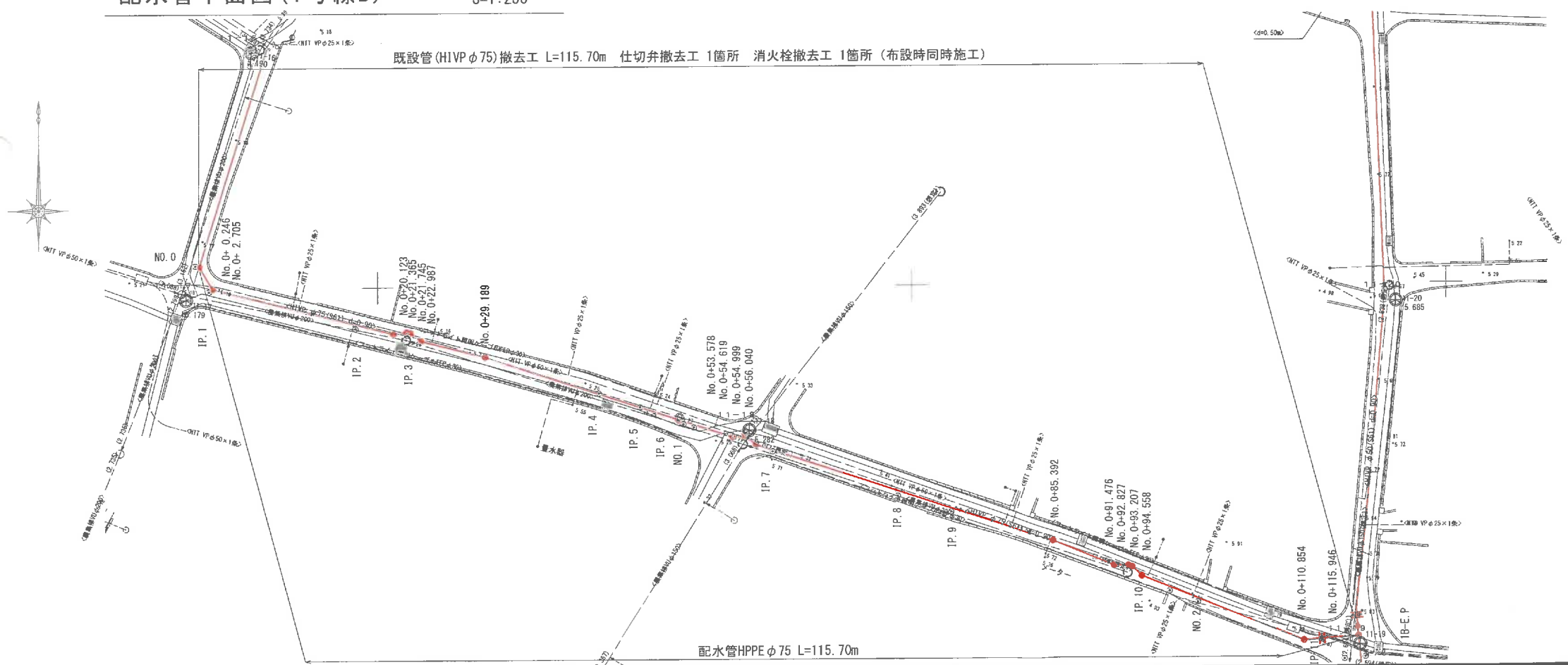
配水管平面図(1号線B)
