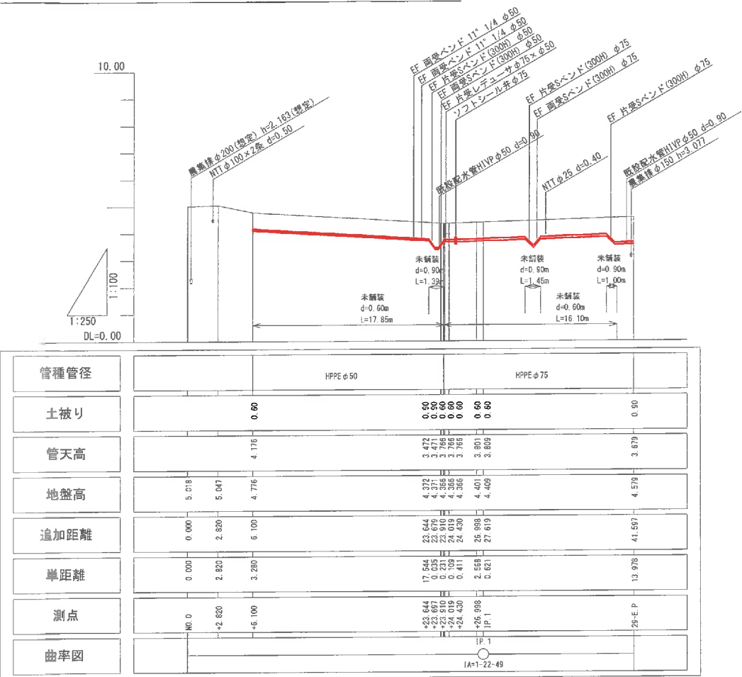
配水管縦断図(29号線)
