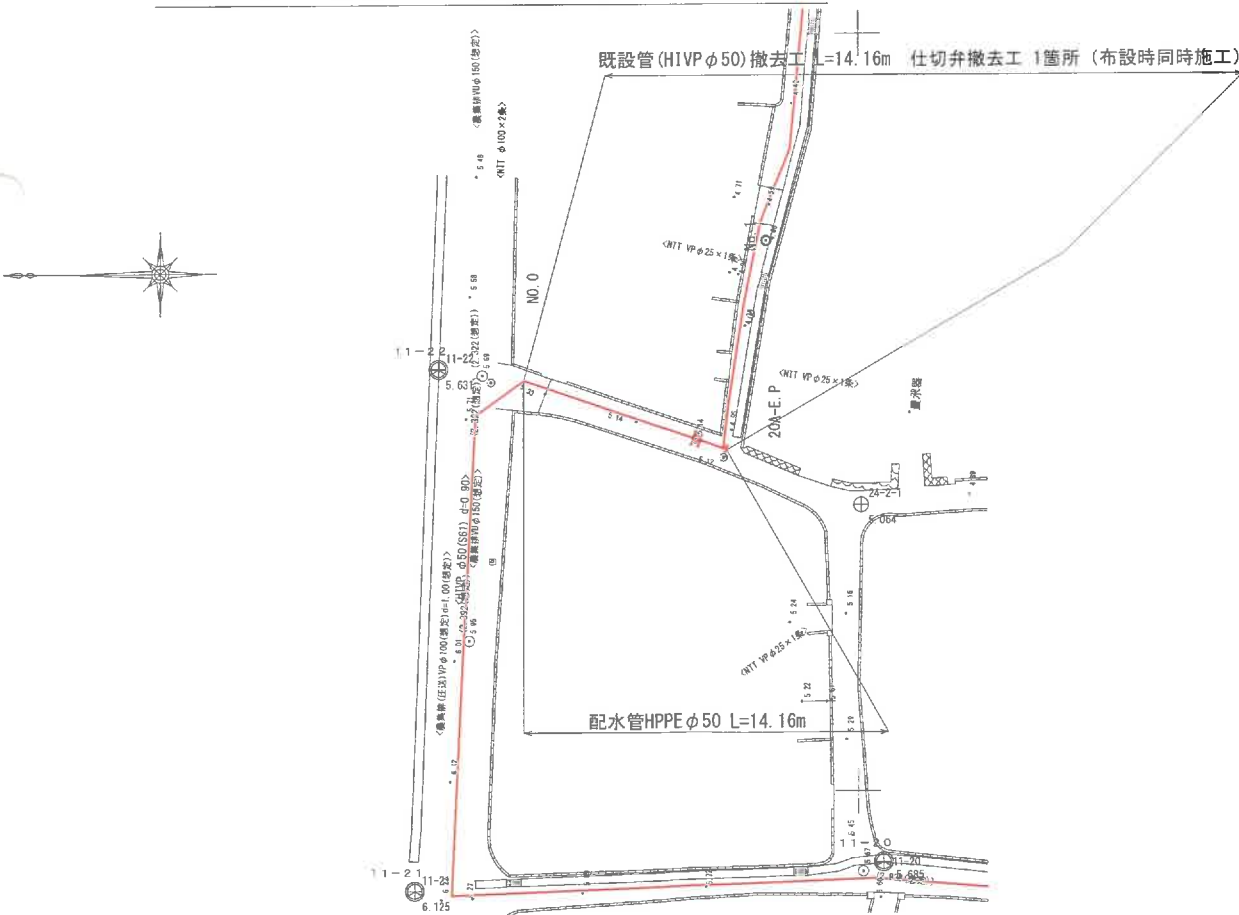
配水管平面図(20号線A) S=1:250
