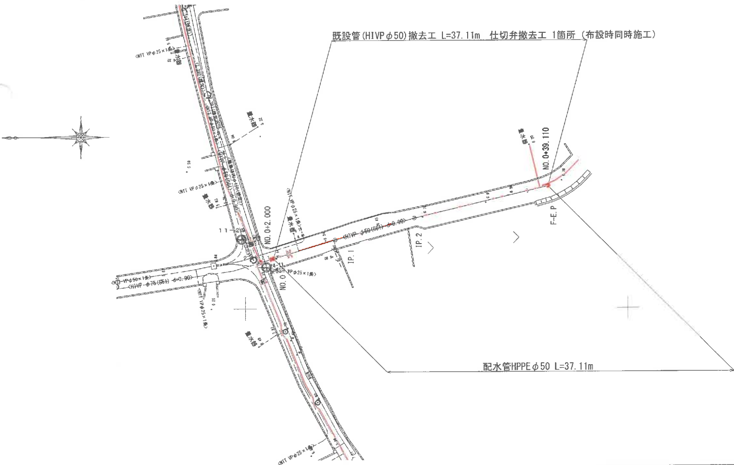
配水管平面図(F路線) S=1:250
