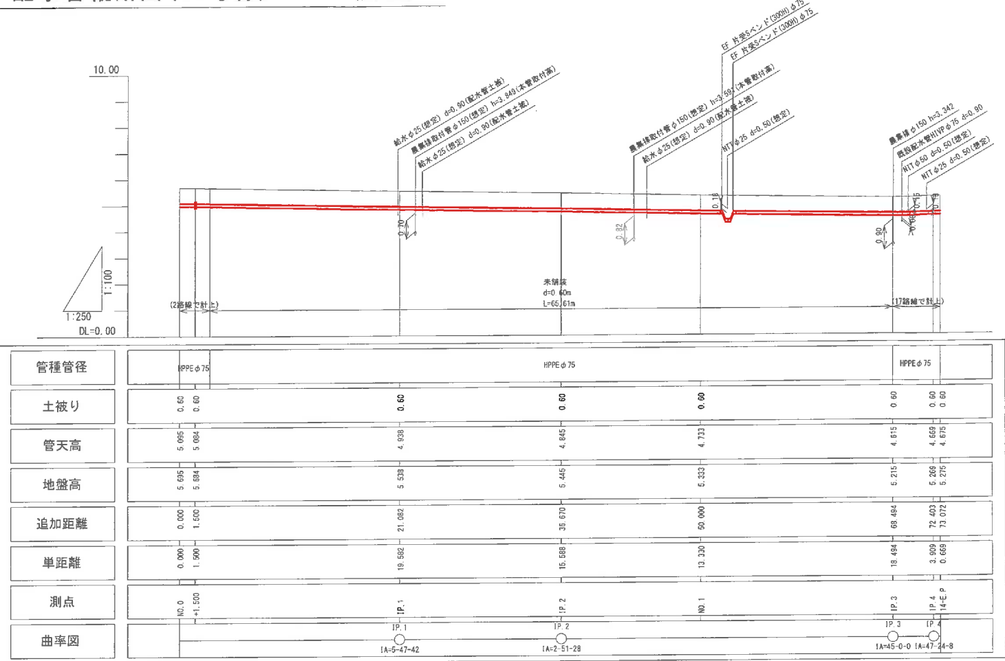
配水管縦断図(14号線) V=1:100 H=1:250
