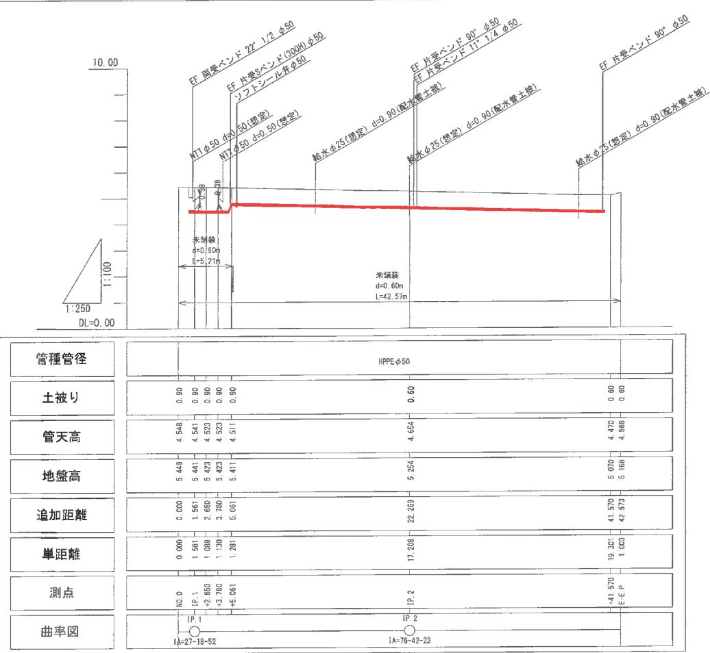
配水管縦断図(E路線) V=1:100 H=1:250
